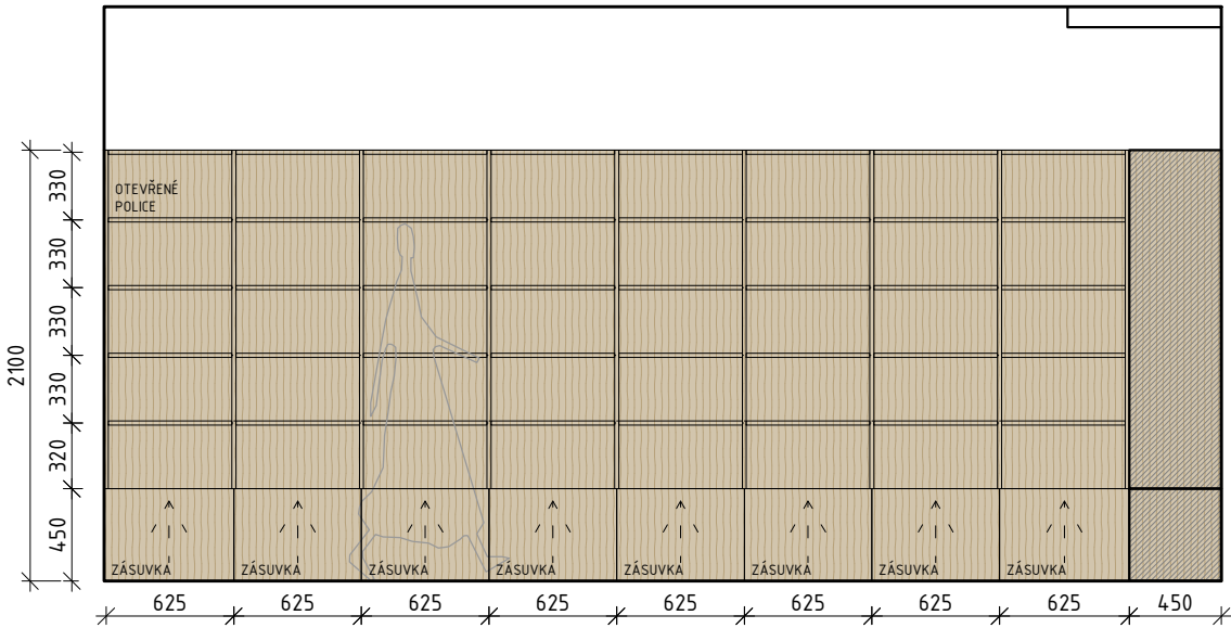
POHLED D
