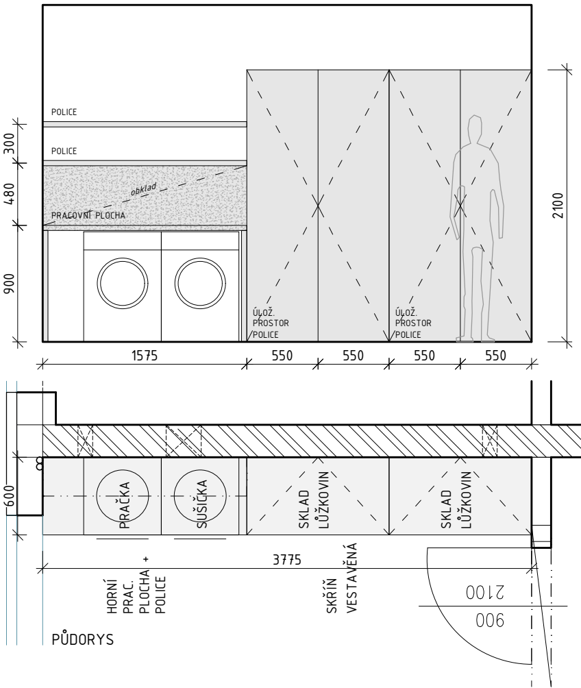
POHLED - zavřené skříně
