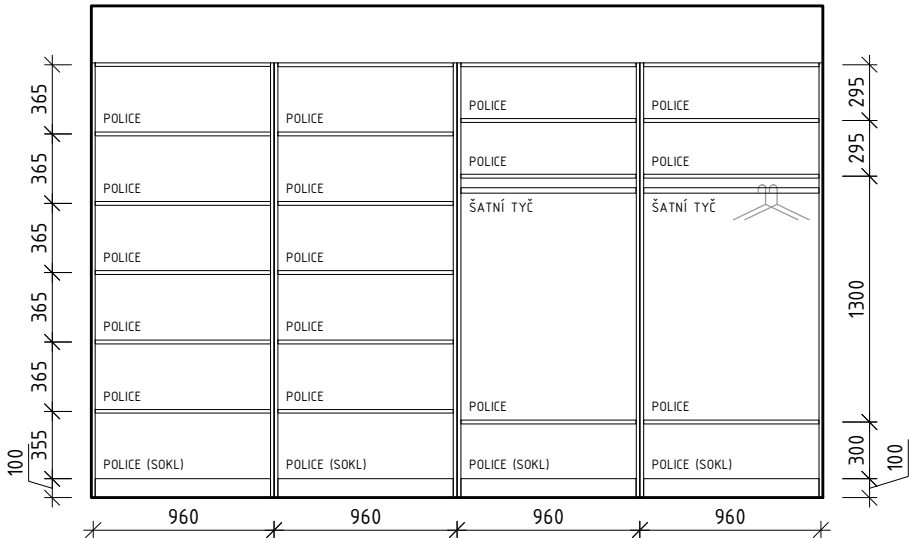
POHLED - otevřené skříně
