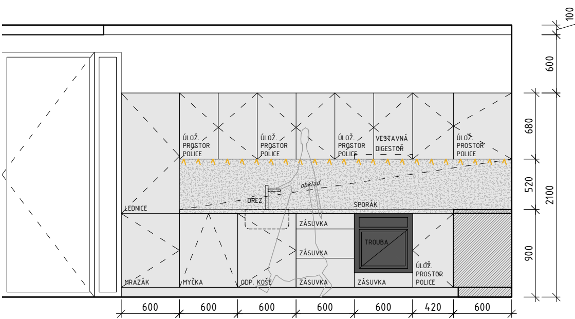
POHLED B
