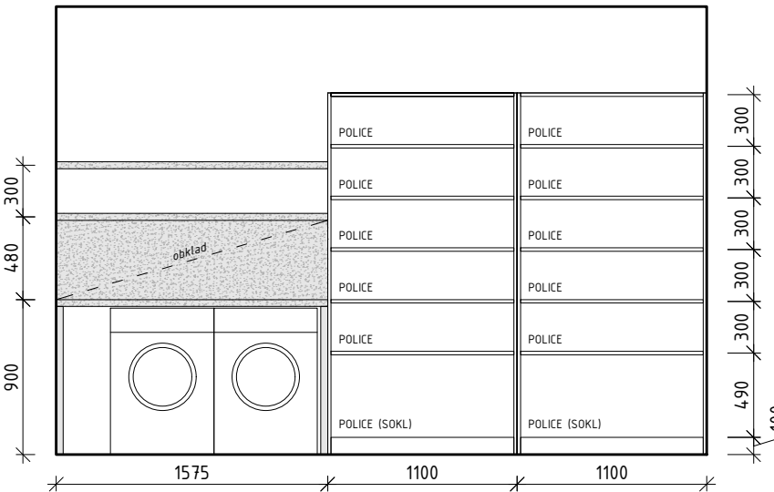
POHLED - otevřené skříně
