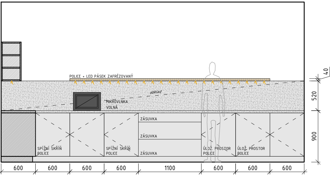
POHLED B
