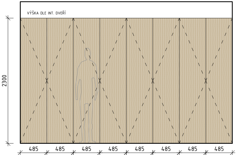
POHLED - zavřené skříně
