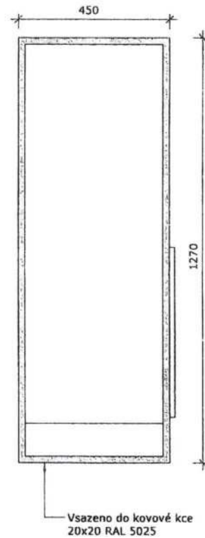
BOČNÍ POHLED
