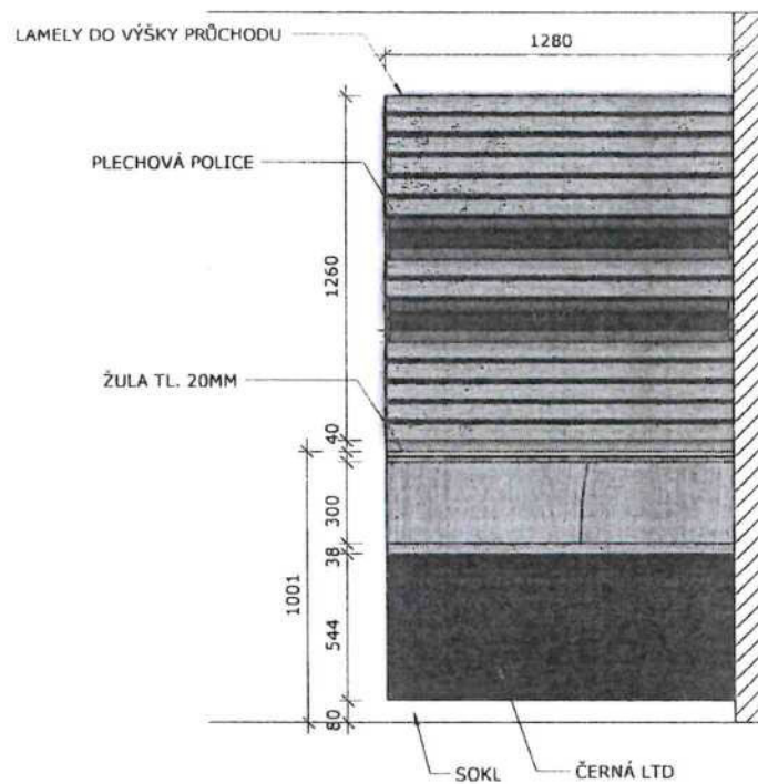
ČELNÍ POHLED
