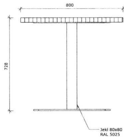
BOČNÍ POHLED
