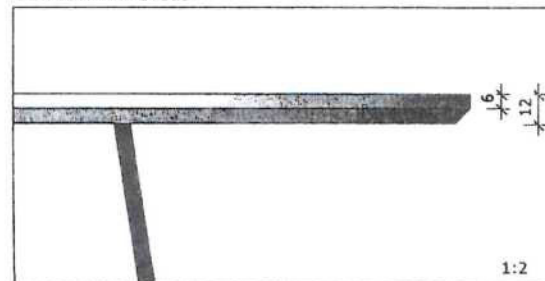
DETAIL HRANY STOLU
