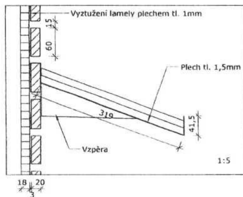
DETAIL ZASUNUTÍ POLICE
