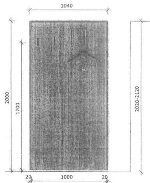
ČELNÍ POHLED
