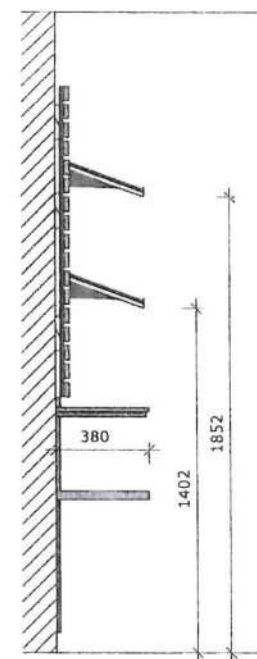
BOČNÍ POHLED
