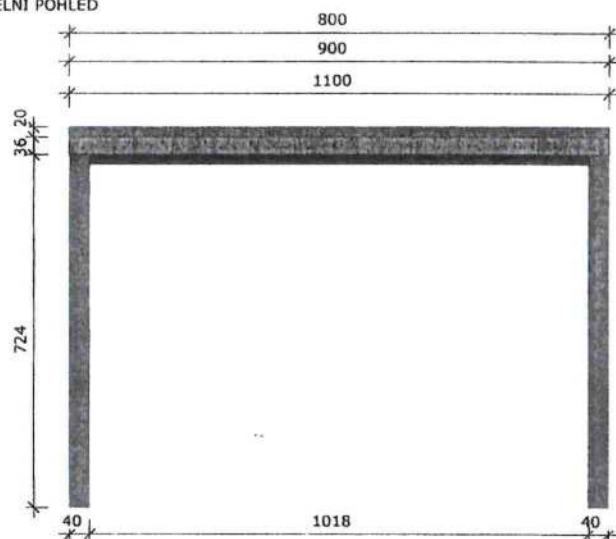
ČELNÍ POHLED
