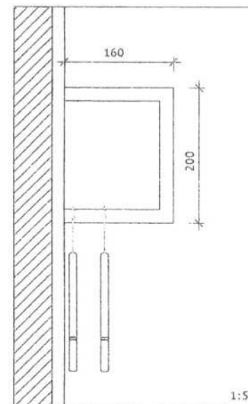
DETAIL ZAVĚŠENÍ RAMÍNEK
