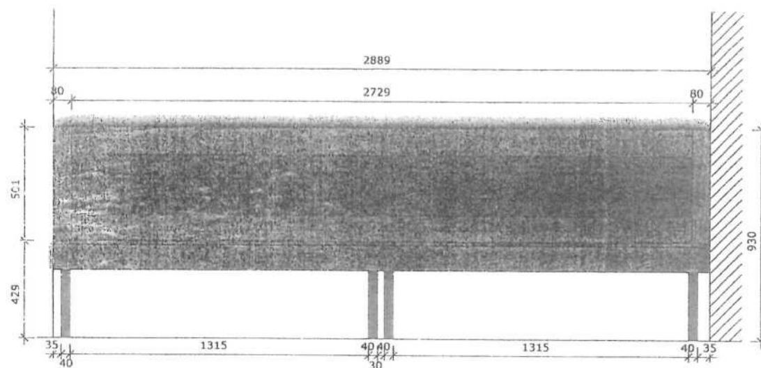
ČELNÍ POHLED
