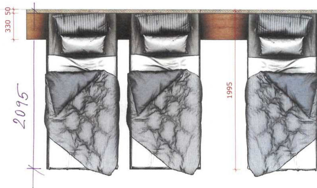
POHLED SHORA
