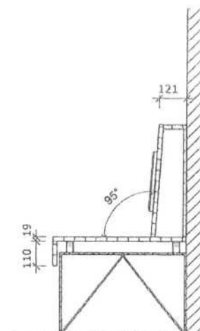
BOČNÍ ŘEZ
