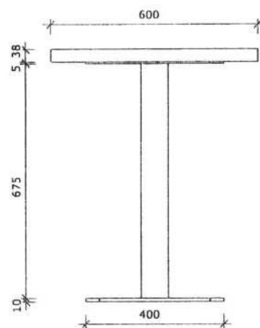
ČELNÍ POHLED
