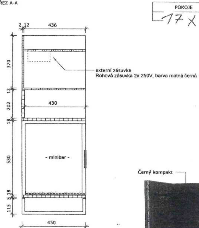
ŘEZ A-A
