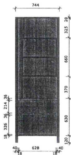
ČELNÍ POHLED
