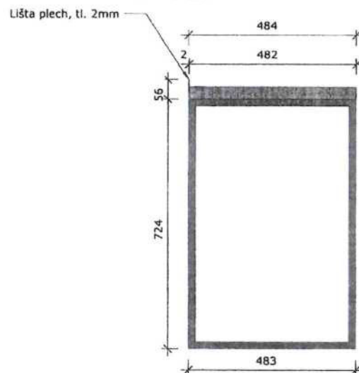
BOČNÍ POHLED
